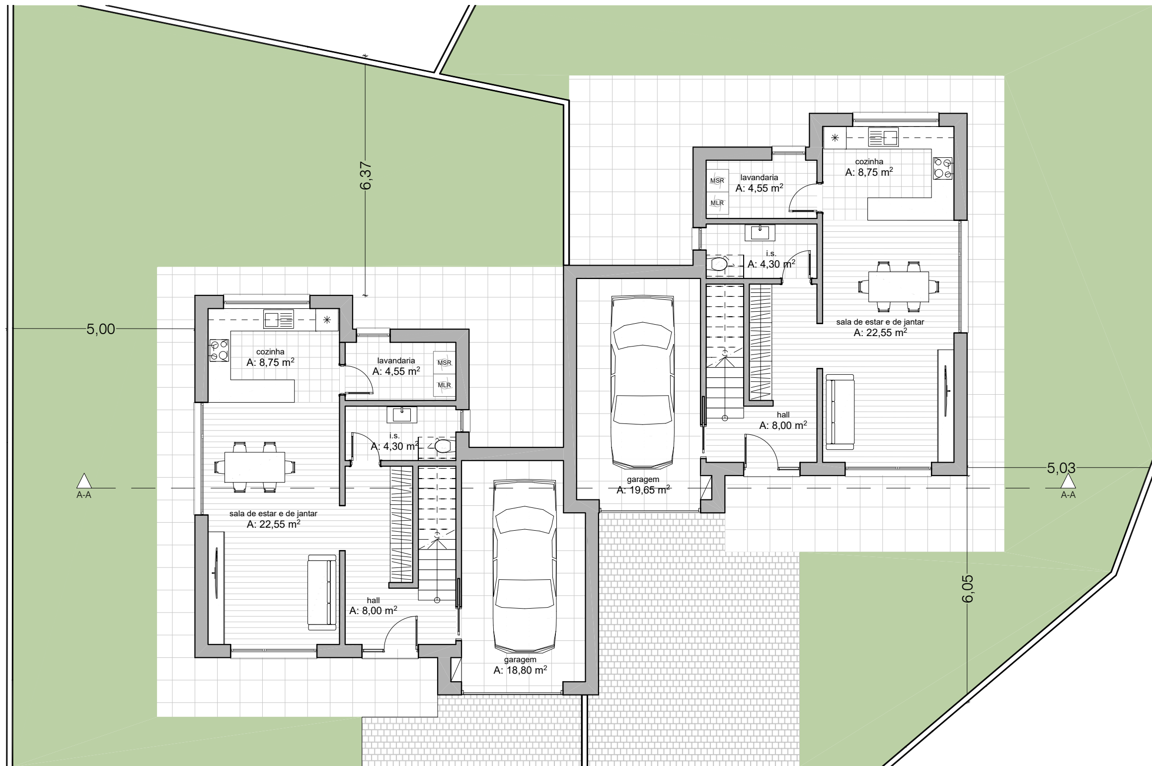
PLANTA DO RÉS DO CHÃO
